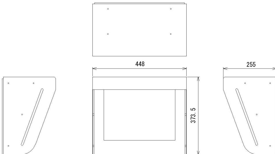
外形寸法図／モニタカバー本体&遮光板
