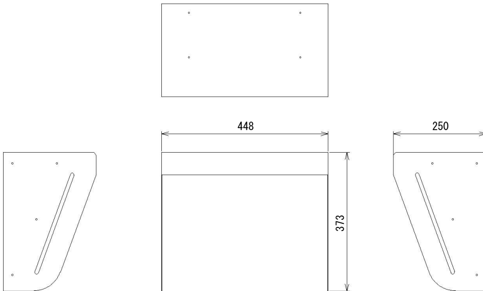
外形寸法図／遮光板 NM-CAF170
