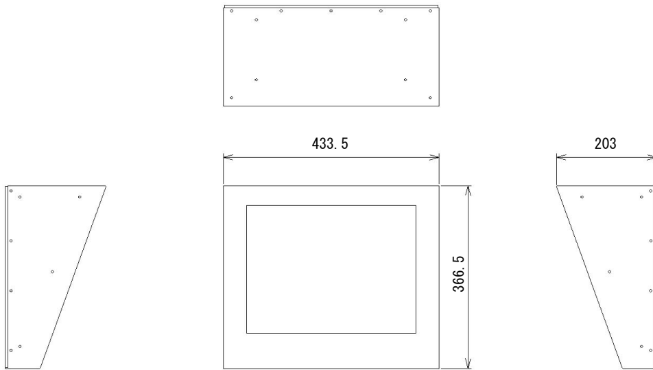
外形寸法図／モニタカバー本体 NM-CAG170-20
